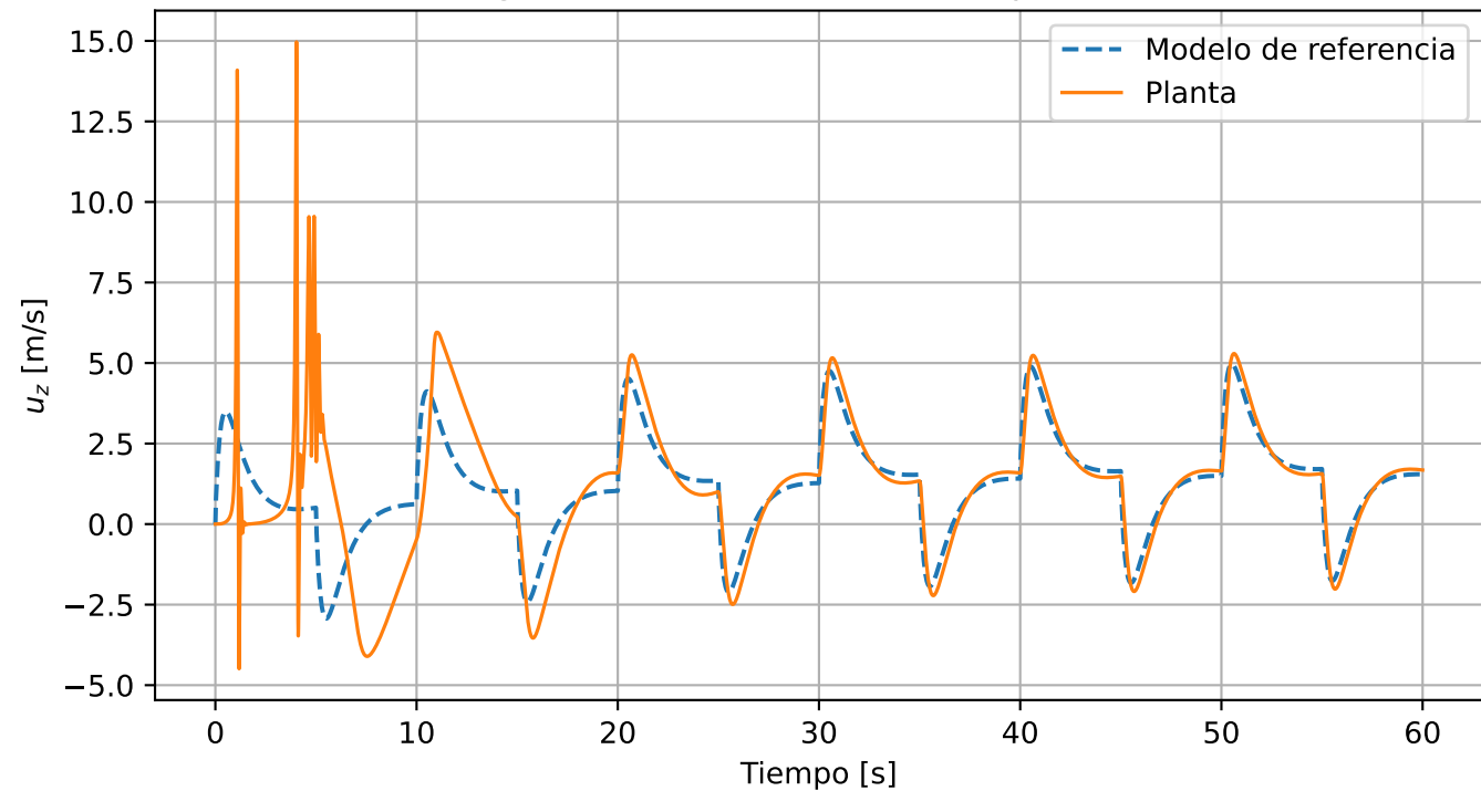
Seguimiento MRAC con tren de pulsos: u_z
